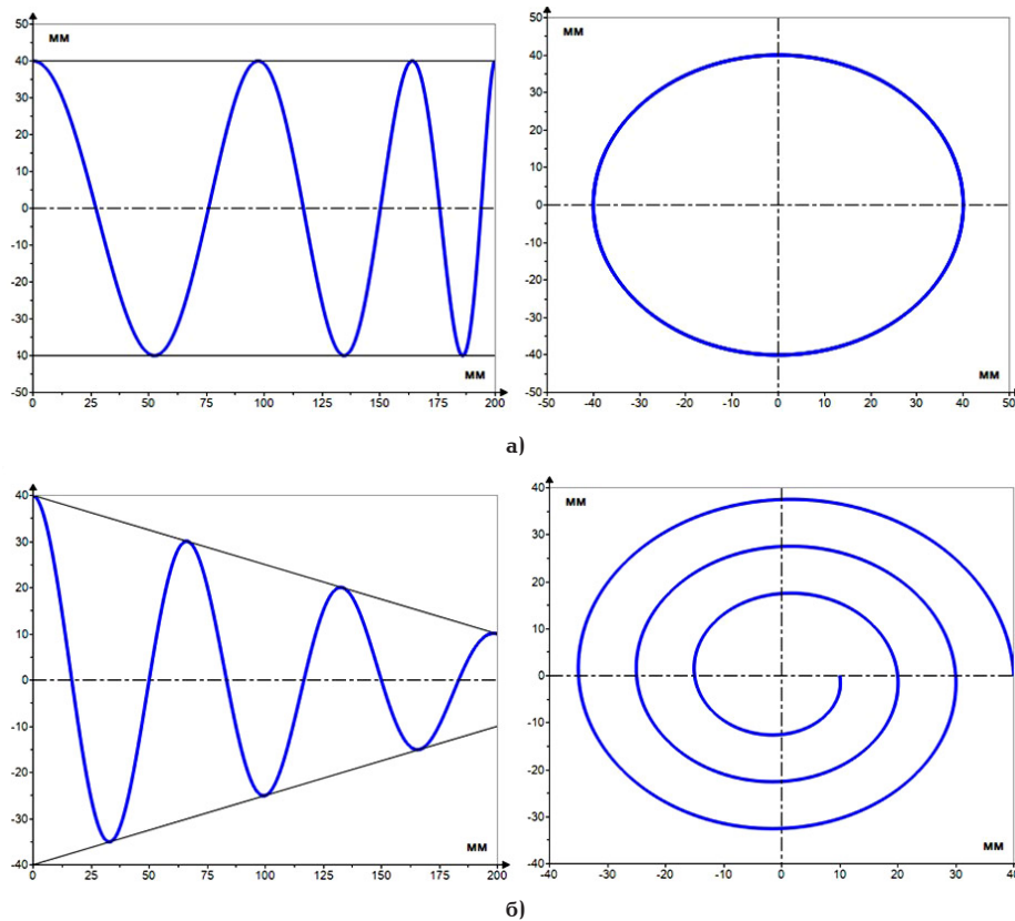
Рис. 5. Винтовые образующие: а — постоянный профиль и переменный шаг винтов; б — переменный профиль и постоянных шаг винтов
