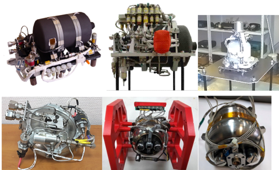
Рис. 6. Двигательные установки для спутниковых платформ различной размерности
