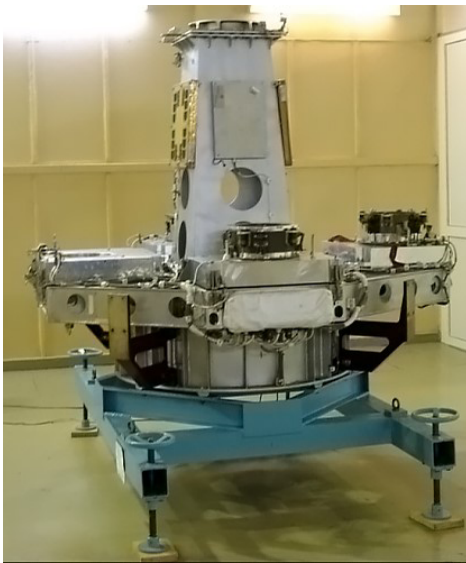
Рис. 2. Адаптер для группового запуска КА на РН «Космос-3М»
