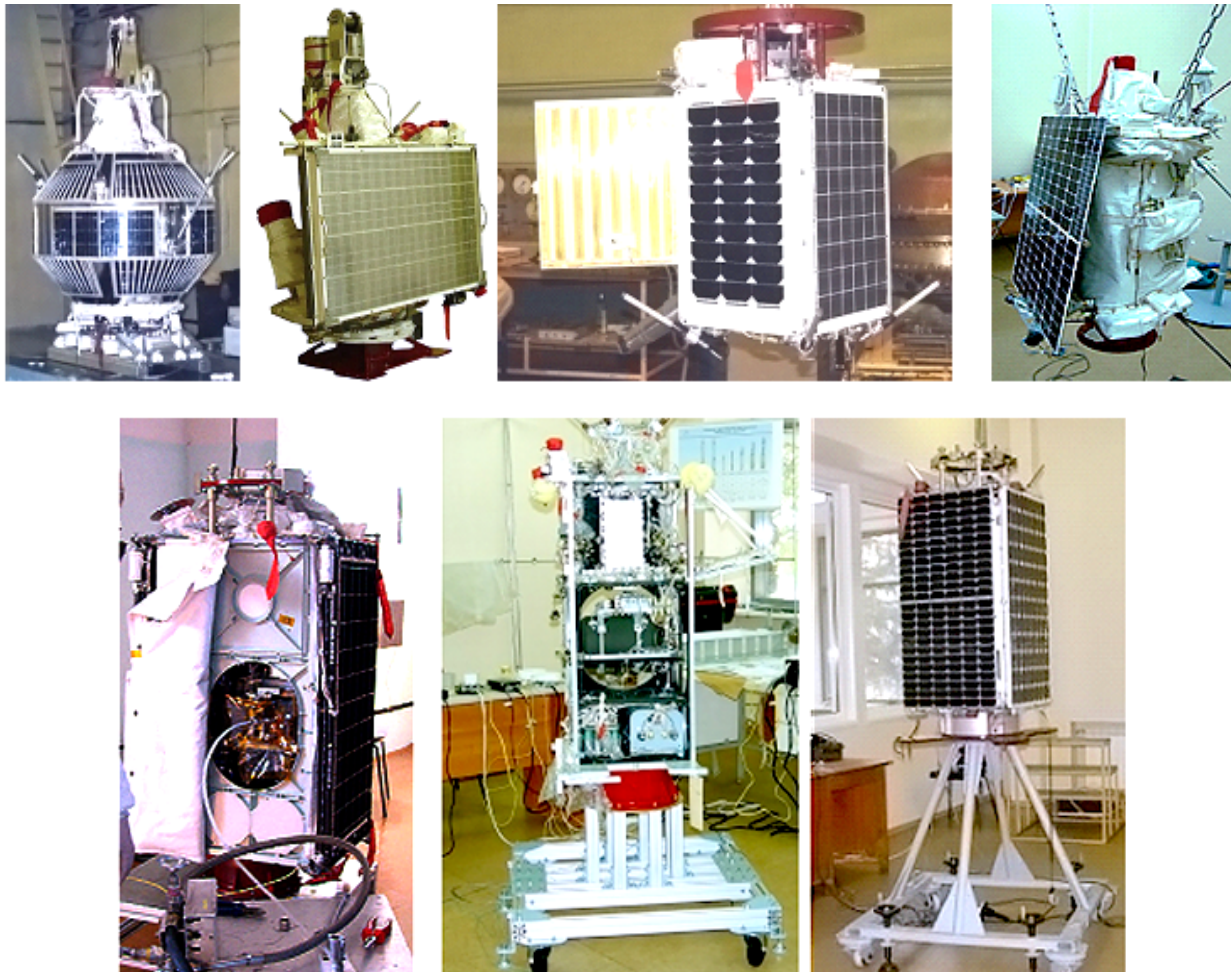
Рис. 3. Малые космические аппараты разработки КБ «Полет»
